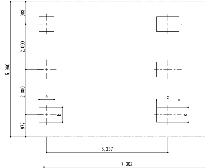
■ 基礎配置図
